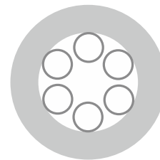
负曲率
